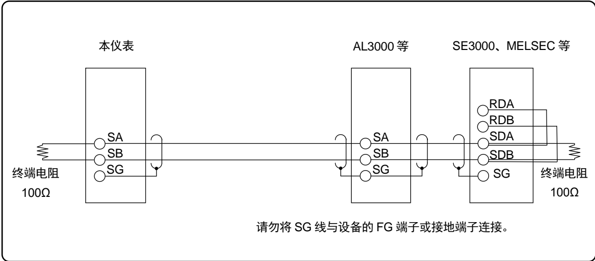
接线示例 1
