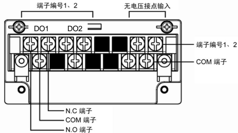
继电器报警输出(2点c接点)
