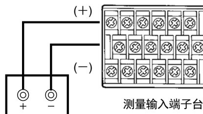
直流标准电压发生器
